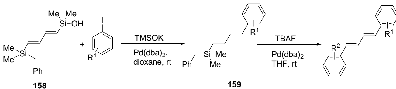
Scheme 63. Hiyama coupling of 1,4-bissilylbutadienes
